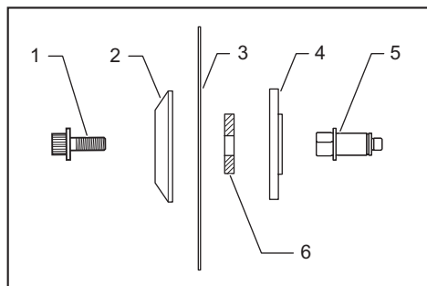
► 1. Perno de cabeza hexagonal 2. Brida exterior 3. Disco de la sierra 4. Brida interior 5. Eje 6. Anillo
