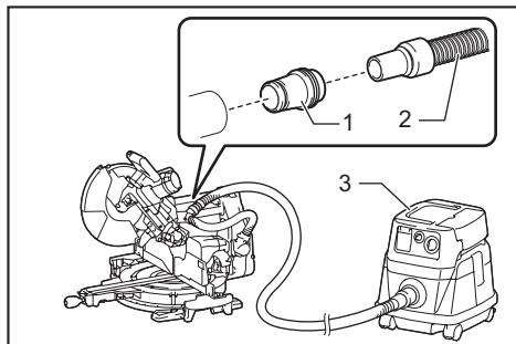
► 1. Manguitos delanteros 24 2. Manguera 3. Aspiradora
