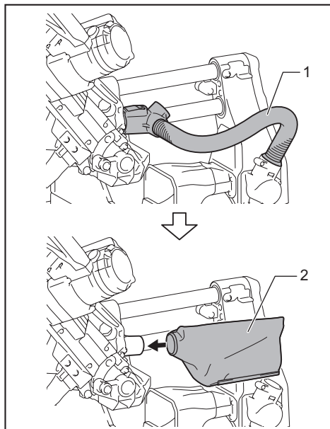
► 1. Manguera de extracción de polvo 2. Bolsa recolectora de polvo
